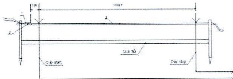
Hình 1 - Sơ đồ đấu nối dây nổ chịu nước để đo tốc độ nổ
